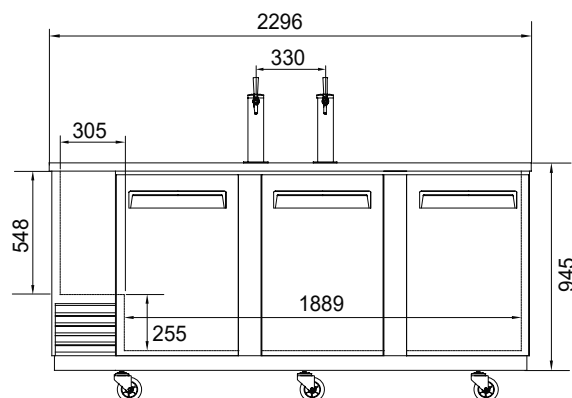
ВИД СПЕРЕДИ
