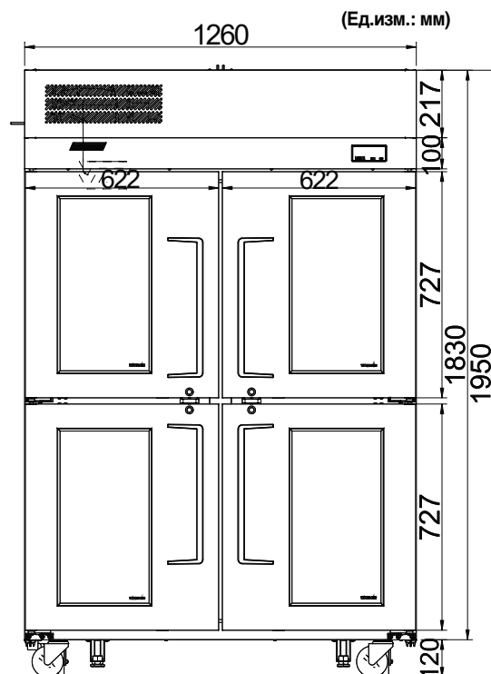
ВИД СПЕРЕДИ
