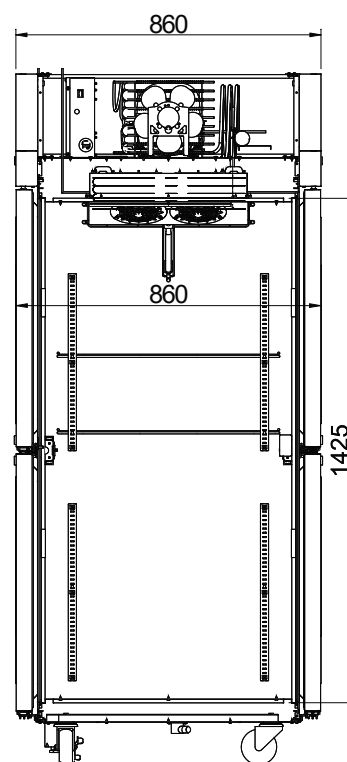
ВИД СБОКУ
