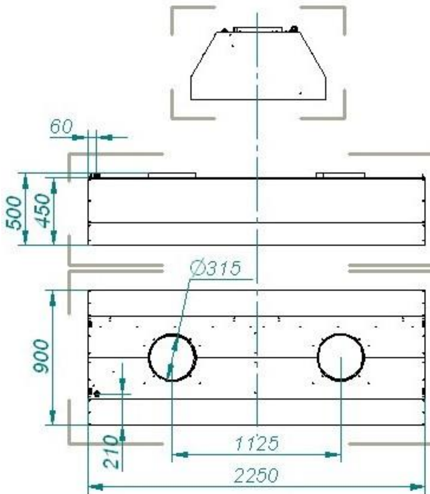
Рис. 3а Зонт вентиляционный ос. пров. 3ВЗ-900-40
