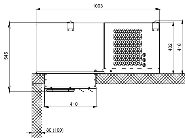
Схема установки холодильной машины в камере
