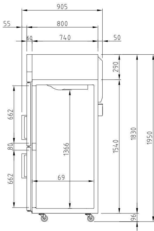
ВИД СБОКУ
