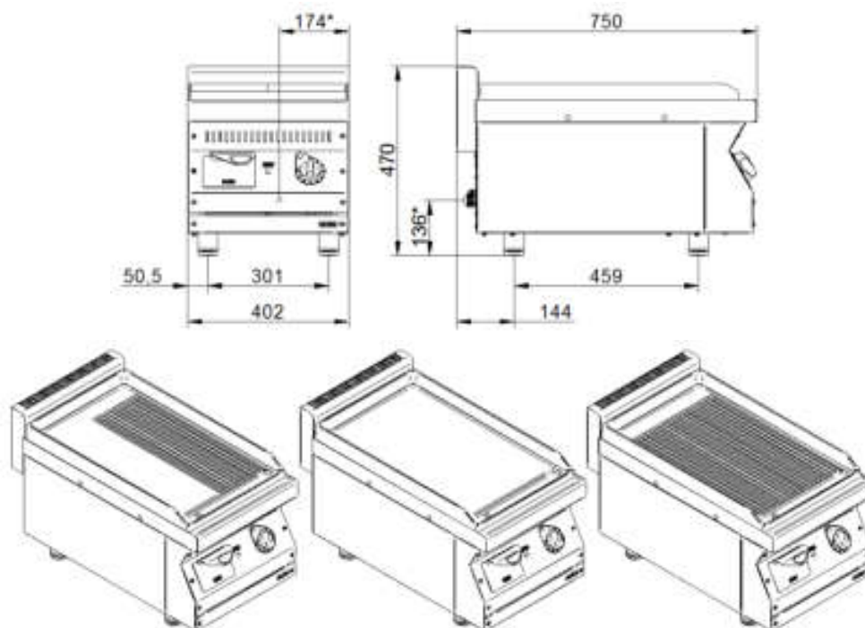
Рис. 1 - Общий вид АКО-40/1Н-Ч-00, АКО-40/1Н-Ч-01, АКО-40/1Н-Ч-02, где * - подвод электропитания
