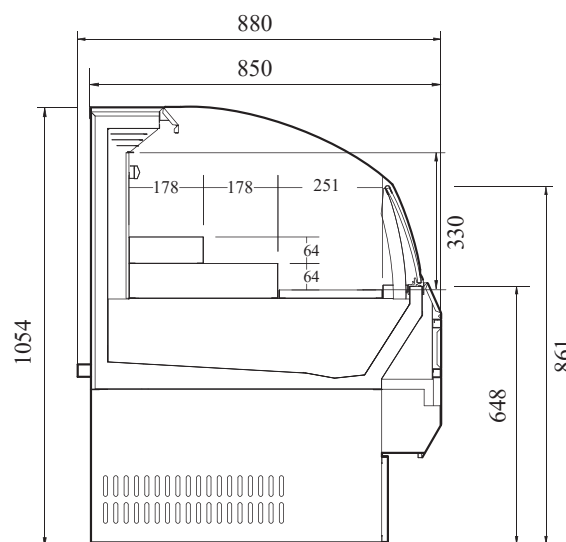
ВИД СБОКУ
