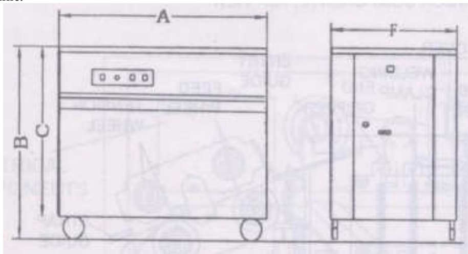
Рис. 13 - Установочные размеры A – 895 мм; B – 735 мм; C – 655 мм; F – 565 мм
