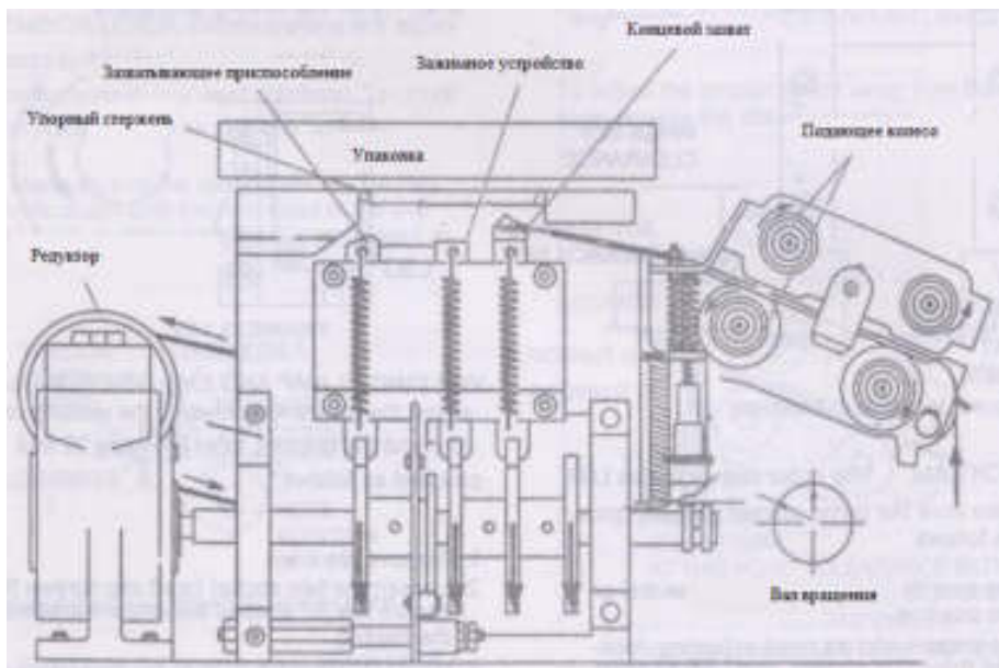
Рис. 11 - Выпуск запаивной ленты; головка в исходном положении, подача ленты
