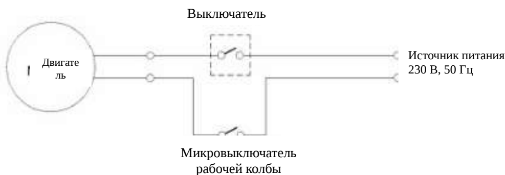
Иллюстрация 6. Схема однофазных электрических соединений на 230 В.
