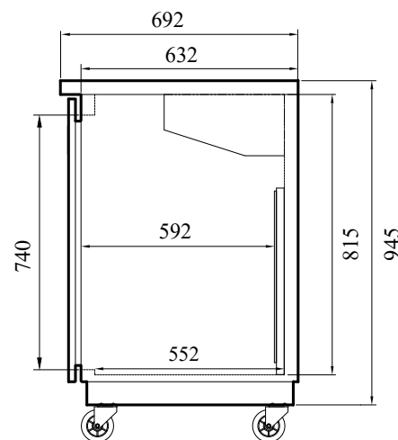
ВИД СБОКУ
