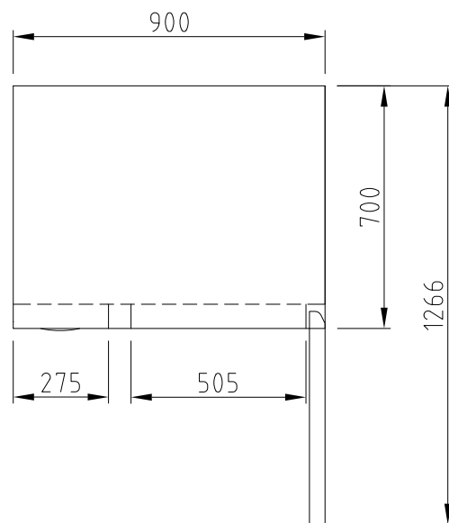
ВИД СВЕРХУ
