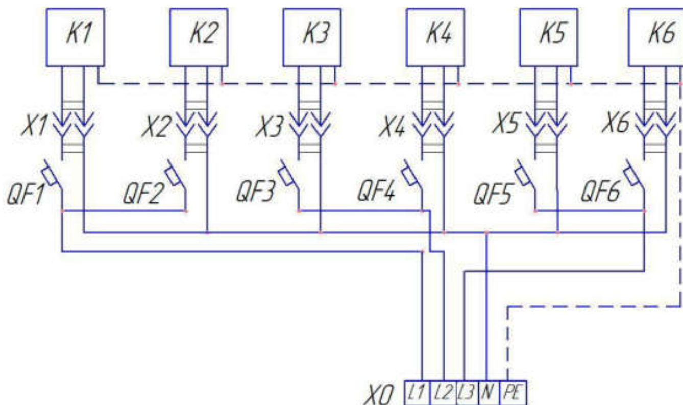
Схема электрическая принципиальная ПЭИ-6D
