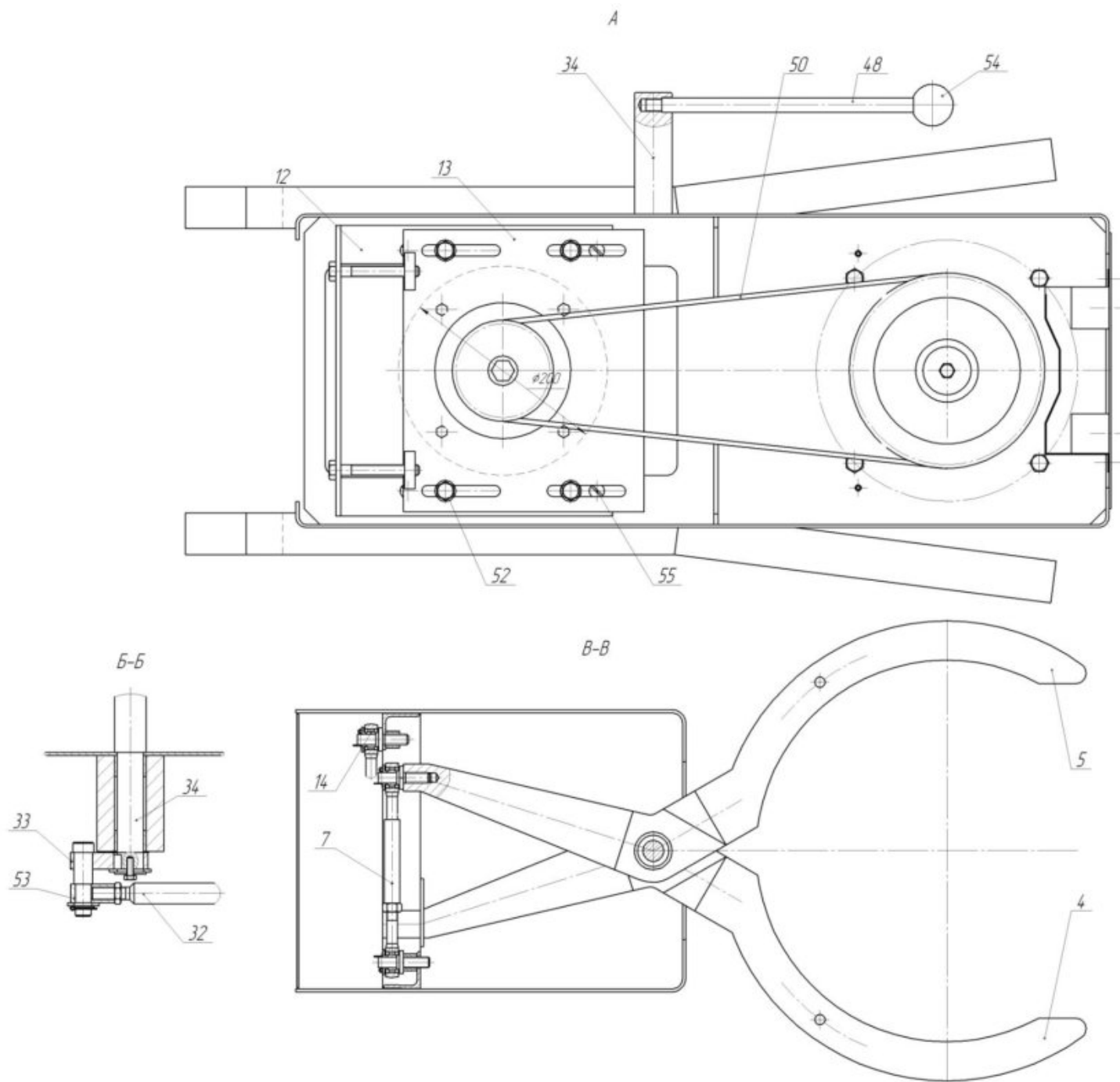
Машина взбивальная МВ-40 (рис.2)
