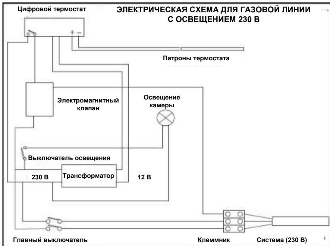
Рисунок 21 – Электрическая схема
