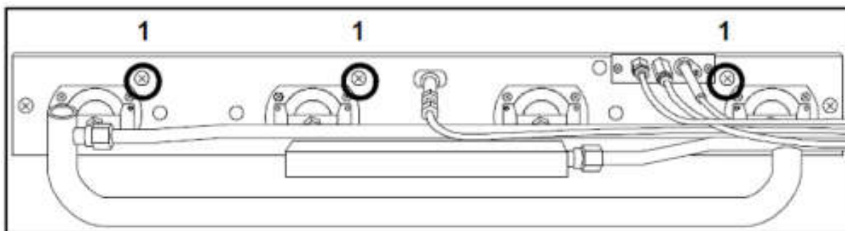
Рисунок 17 – Замена запальной горелки
