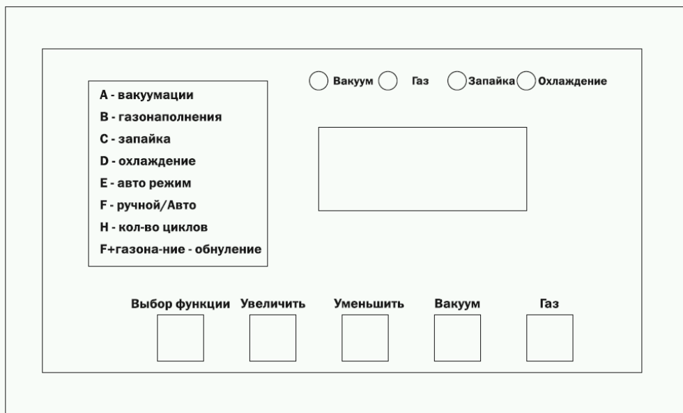
Рис. 1 – Панель управления. Манометр и кнопка Аварийной остановки вынесены с отдельный блок
