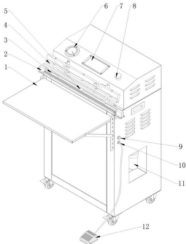
Рис. 2 – Деталировка оборудования (напольная версия)
