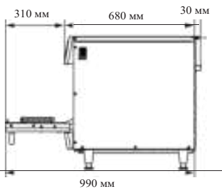
ВИД СБОКУ С ОТКРЫТОЙ ДВЕРЦЕЙ
