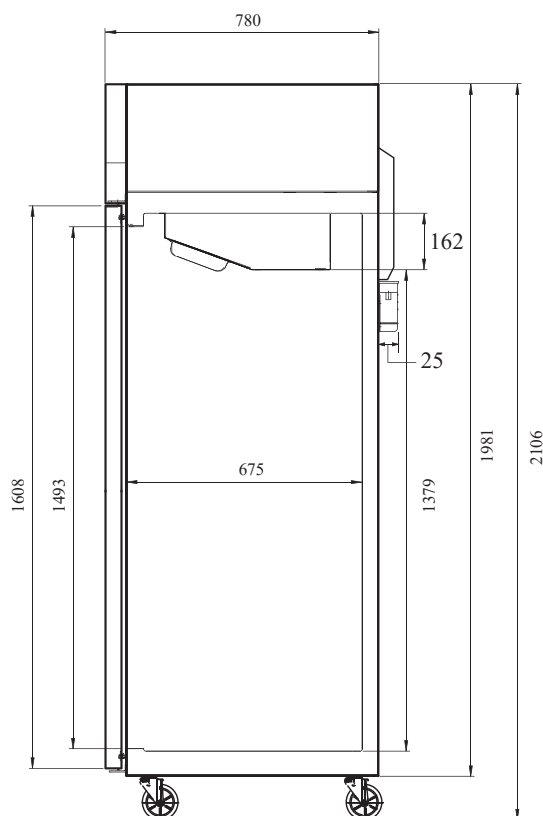
ВИД СБОКУ
