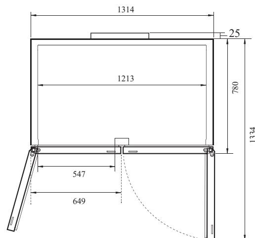
ВИД СВЕРХУ
