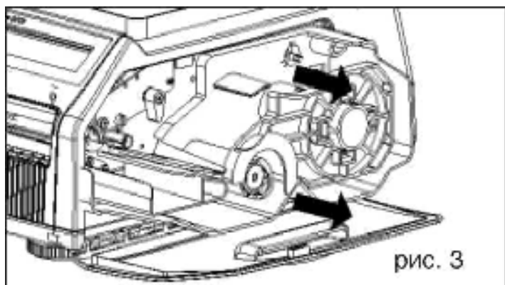
Рисунок 1.13 – Снятие картриджа
