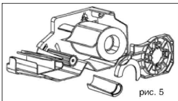
Рисунок 1.15 – Установка рулона
