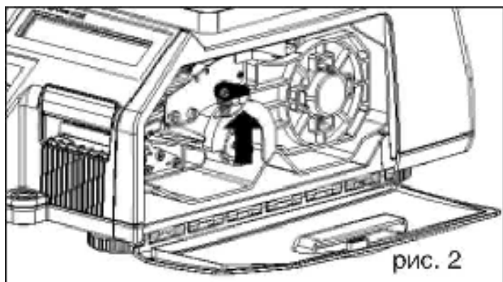
Рисунок 1.12 – Подъем рычага
