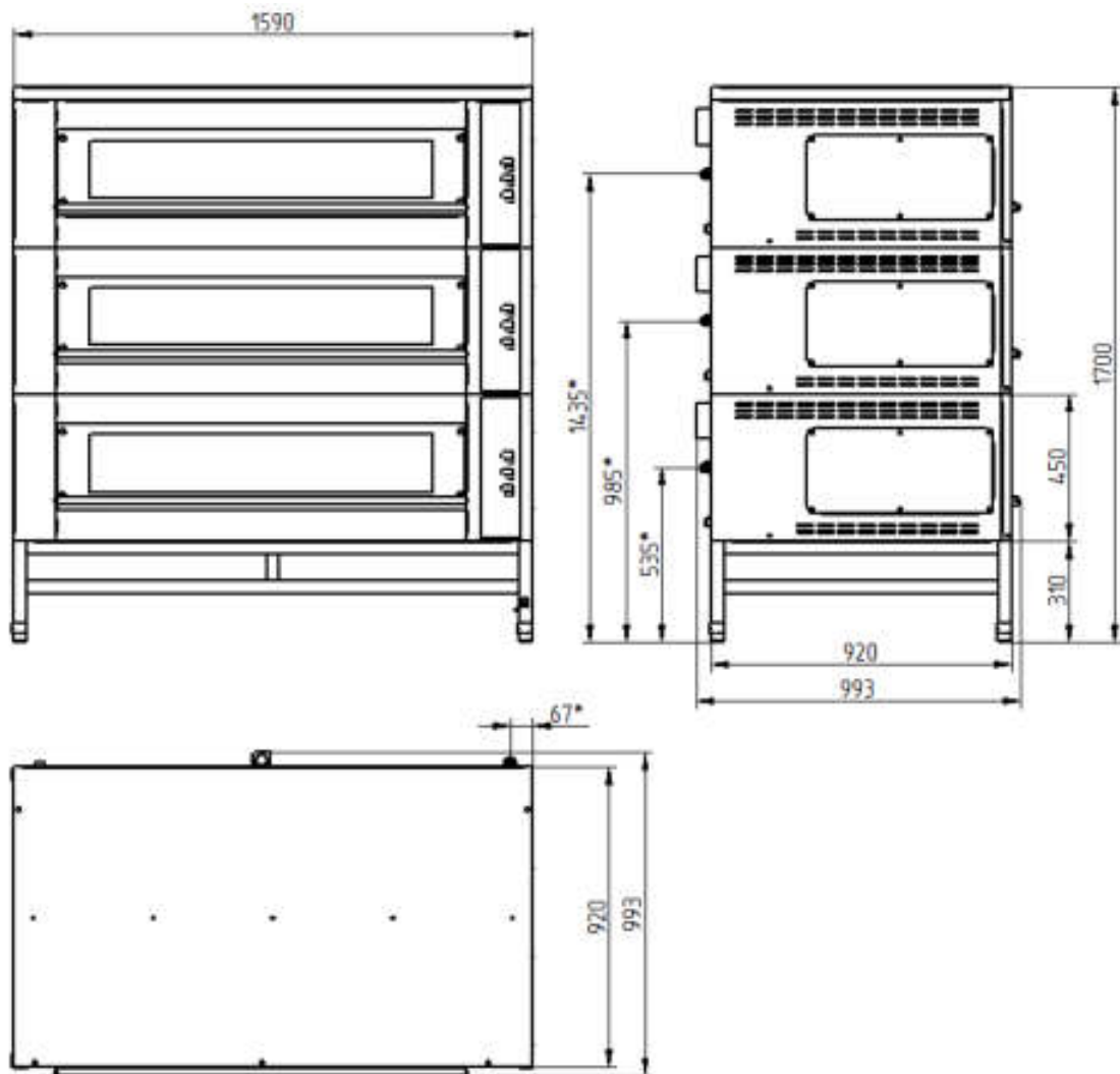
Рис. 1. Общий вид ЭШП-3-01КП 3EN Super.
