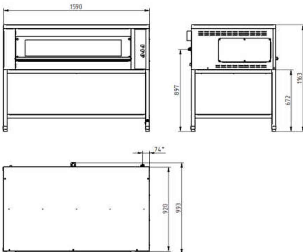
Рис. 2. Общий вид ЭСП-2-01КП 3EN Super.
