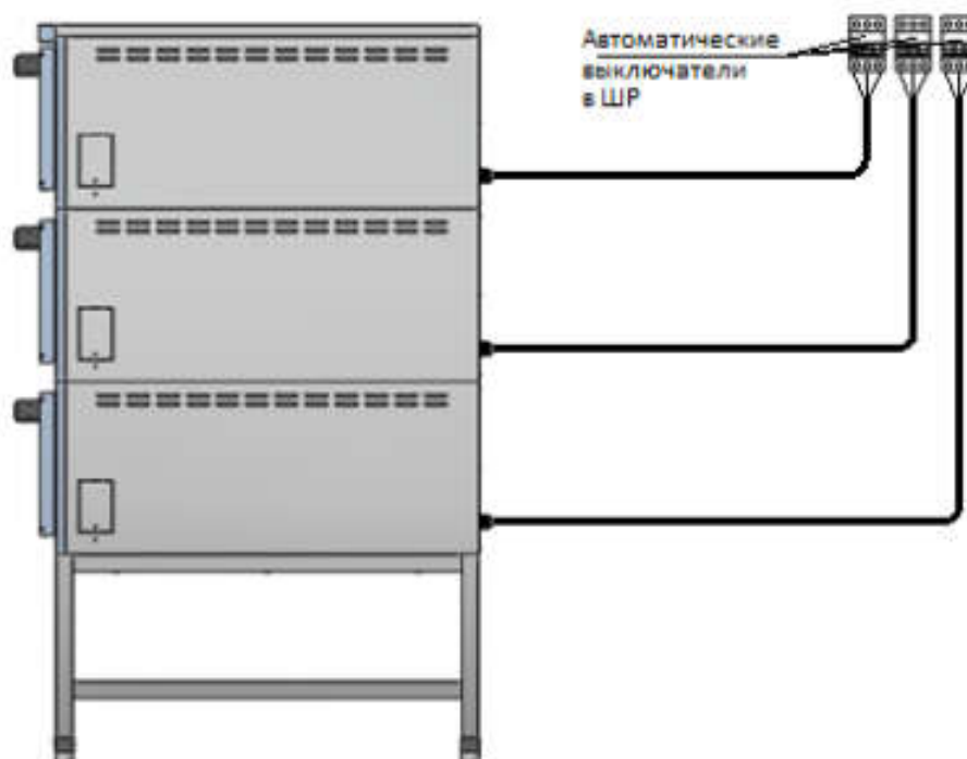
Рис.5 Схема подключения ЭСП-3-01КП 3EN Super к сети
