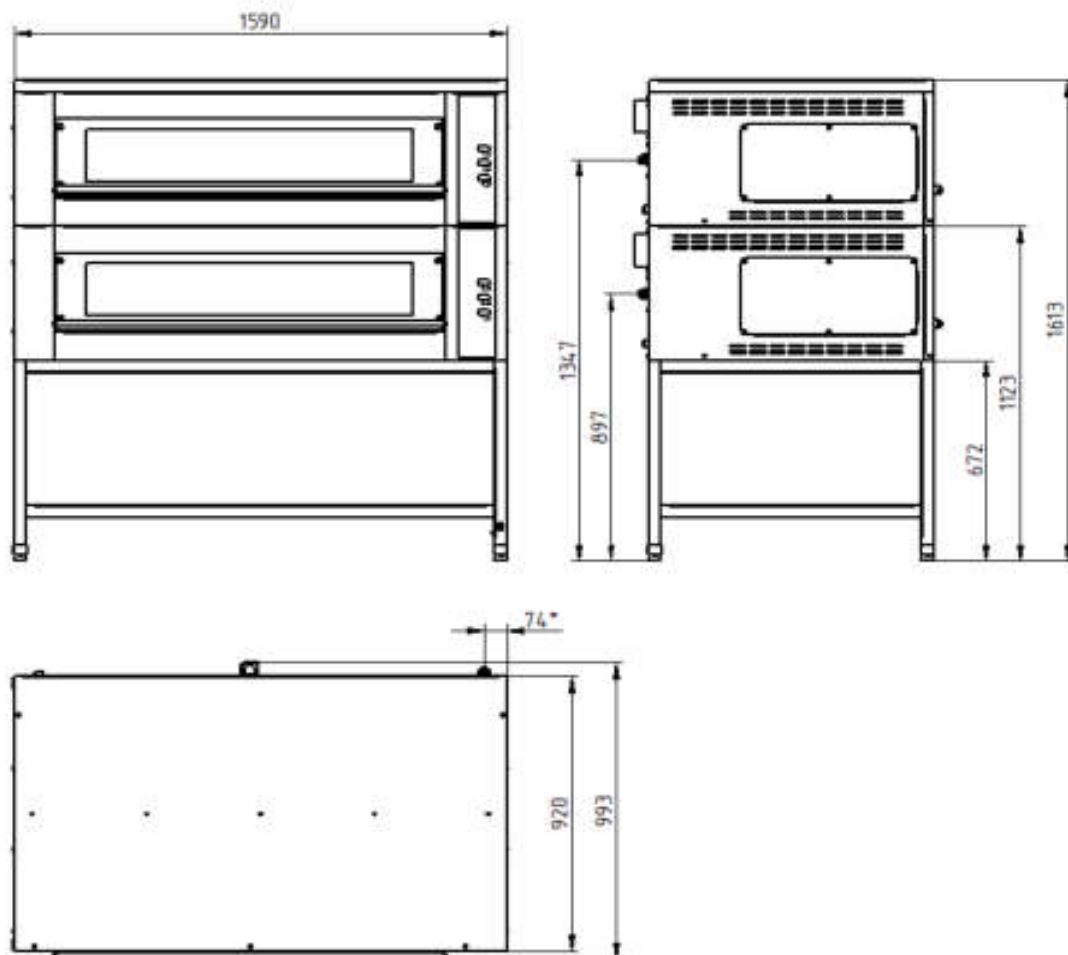
Рис. 2. Общий вид ЭСП-2-01КП 3EN Super.
