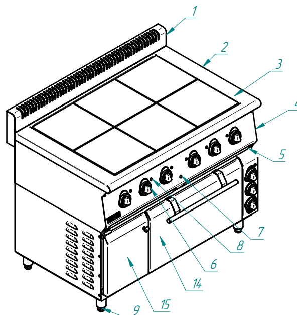
Плита электрическая ПЭ67Ж-02
