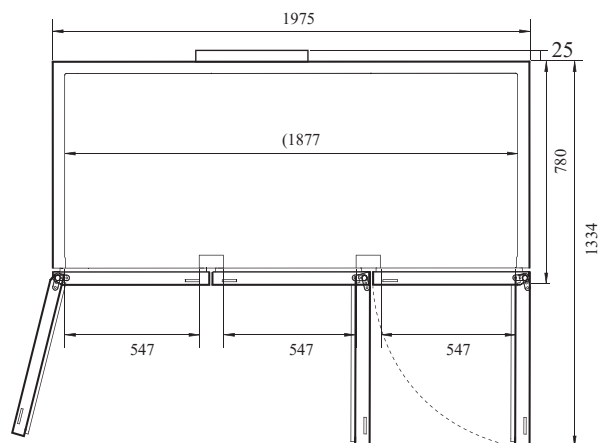
ВИД СВЕРХУ
