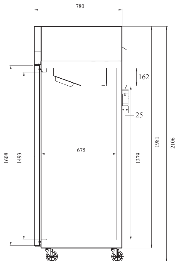
ВИД СБОКУ
