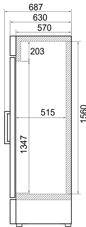
ВИД СБОКУ
