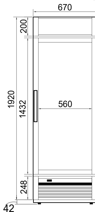
ВИД СПЕРЕДИ
