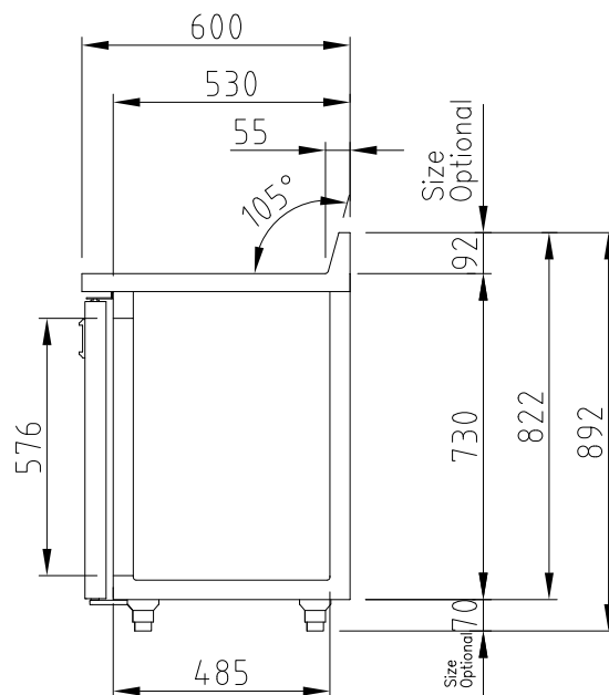
ВИД С БОКУ
