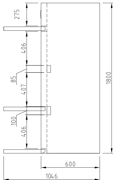
ВИД С ВЕРХУ
