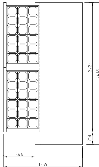
ВИД СВЕРХУ
