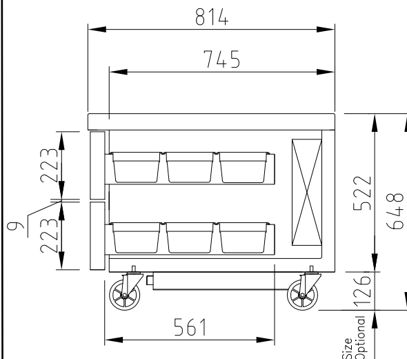
ВИД СБОКУ
