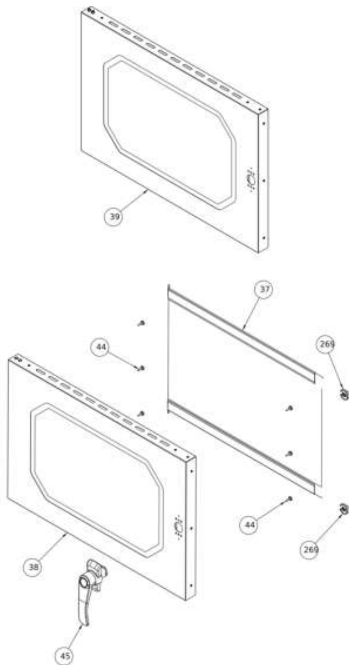
Door
