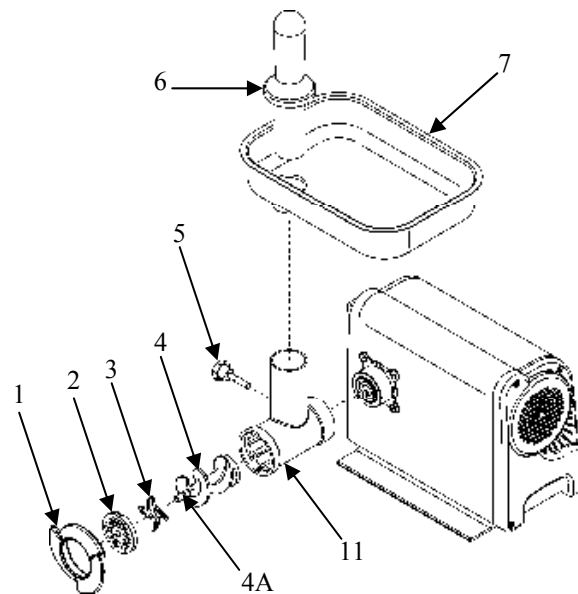
Рис. 10a - Демонтаж компонентов ТС
