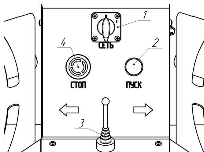
Пульт управления.
