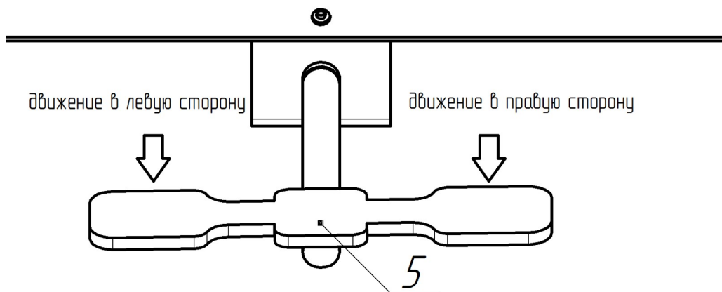
Рукоятка регулировки зазора.
