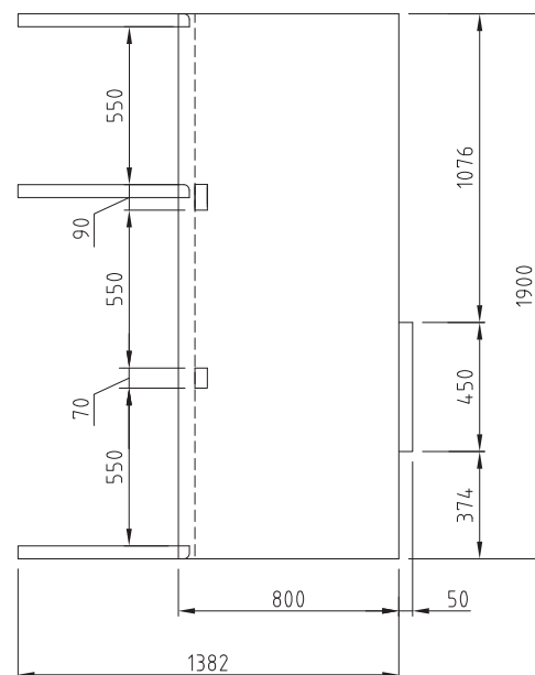
ВИД СВЕРХУ
