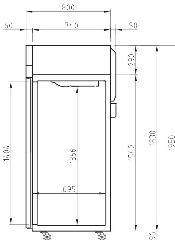
ВИД СБОКУ
