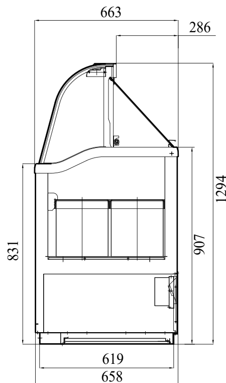
ВИД СБОКУ
