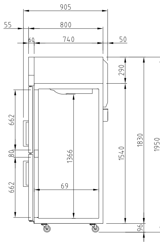
ВИД СБОКУ
