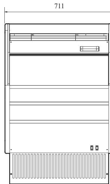
ВИД СПЕРЕДИ
