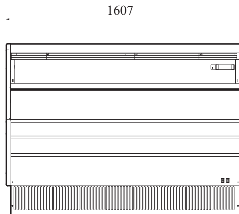
ВИД СПЕРЕДИ
