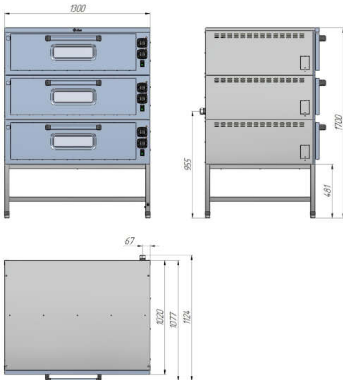
Рис. 1. Общий вид ЭСП-3-01.
