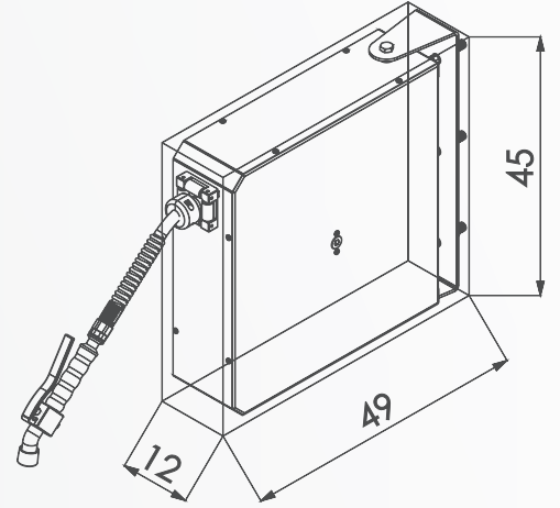
Ürün Kodu: 0904 Ürün Adı: 15 Metre Geri Toplamalı
