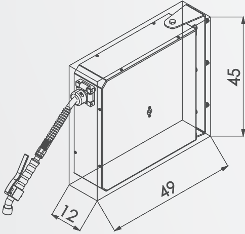
Ürün Kodu: 0902 Ürün Adı: 10 Metre Geri Toplamalı
