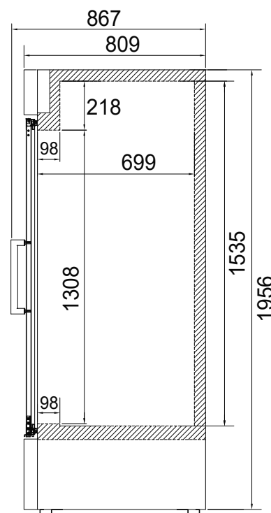
ВИД СБОКУ
