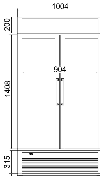
ВИД СПЕРЕДИ
