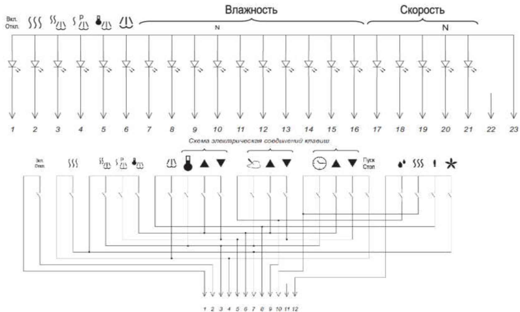
Рис. 11 Схема пленочной клавиатуры
