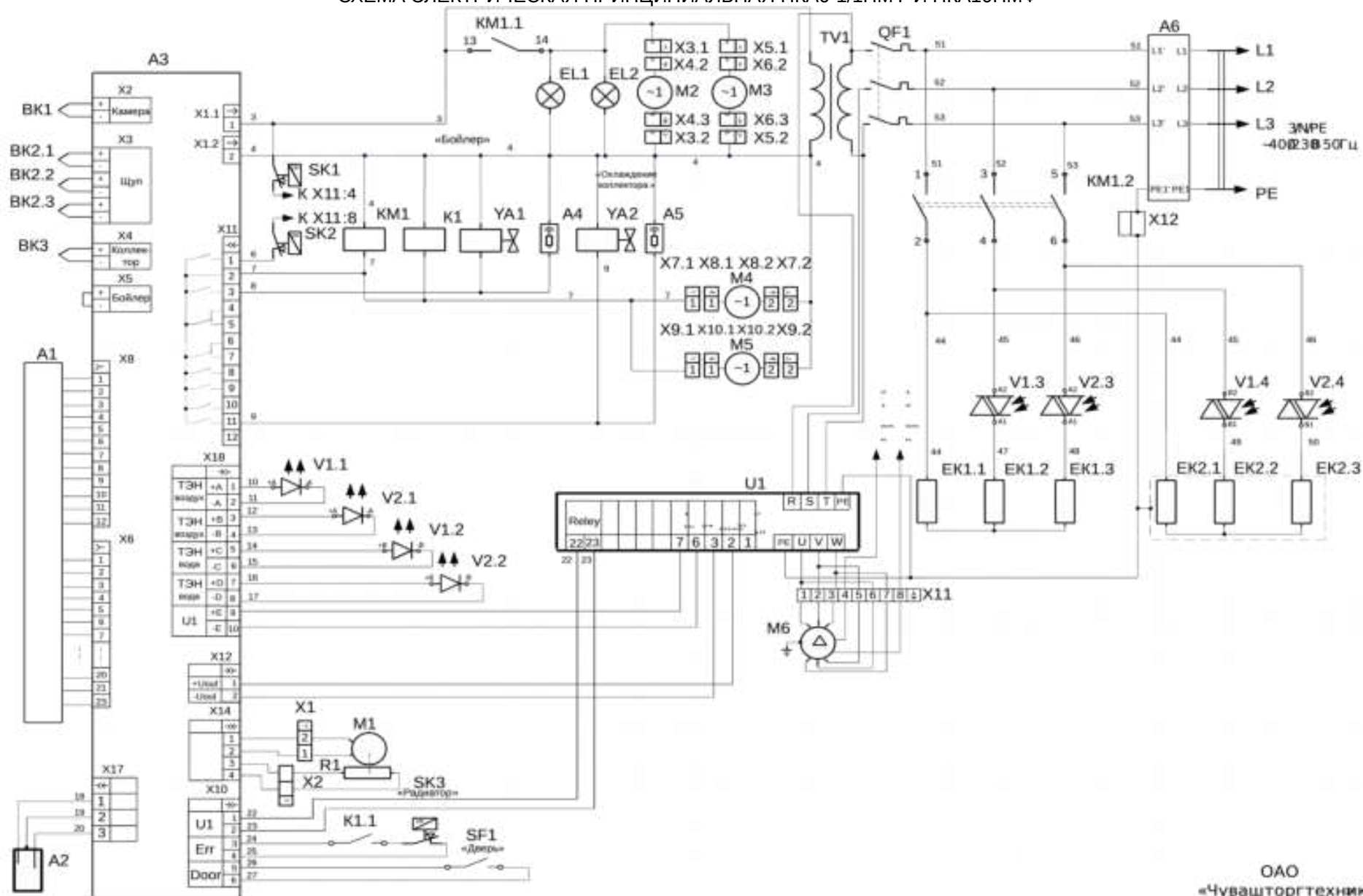
СХЕМА ЭЛЕКТРИЧЕСКАЯ ПРИНЦИПИАЛЬНАЯ ПКА6-1/1ПМФ И ПКА10ПМФ
