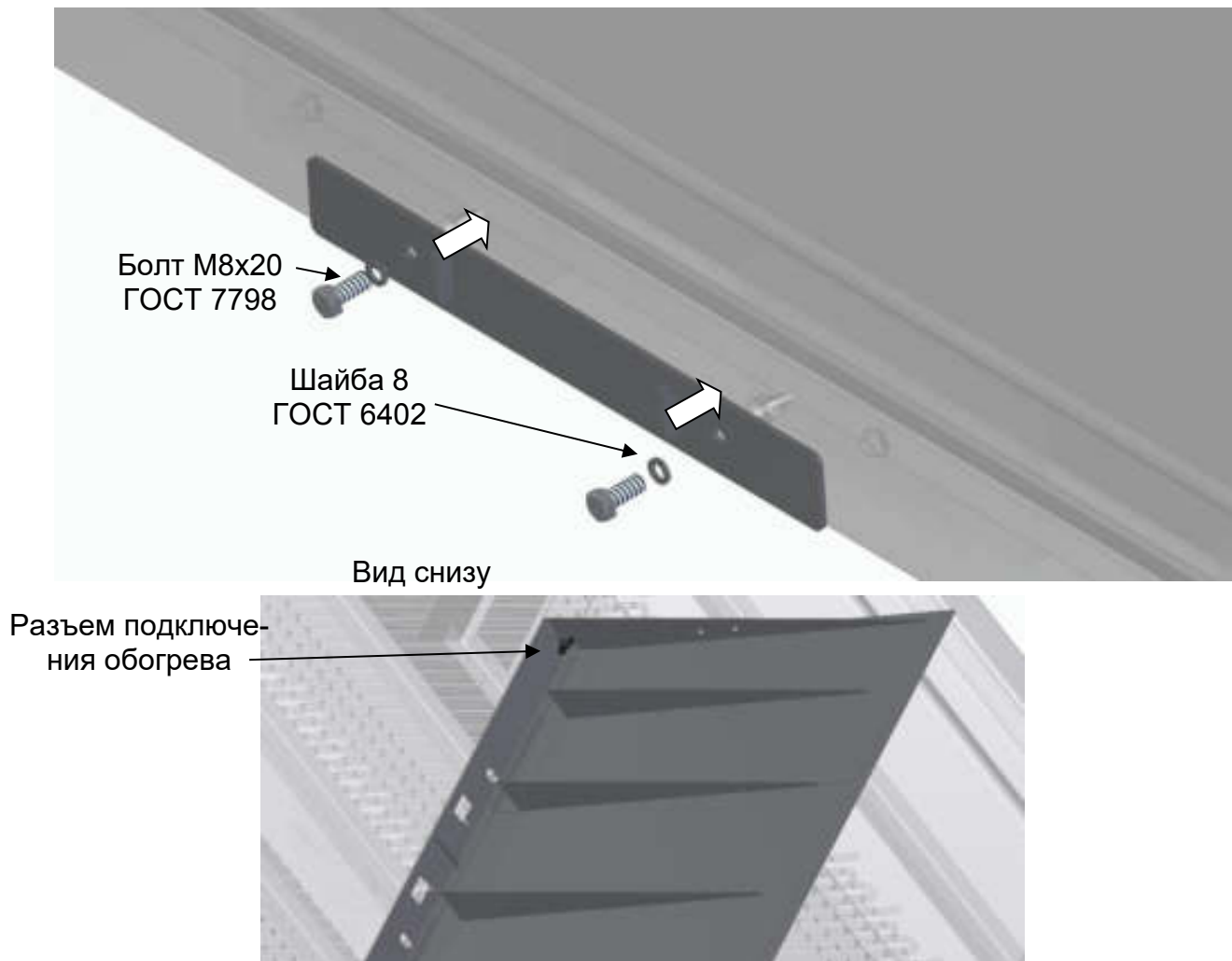
Рис. 25 Установка пандуса
