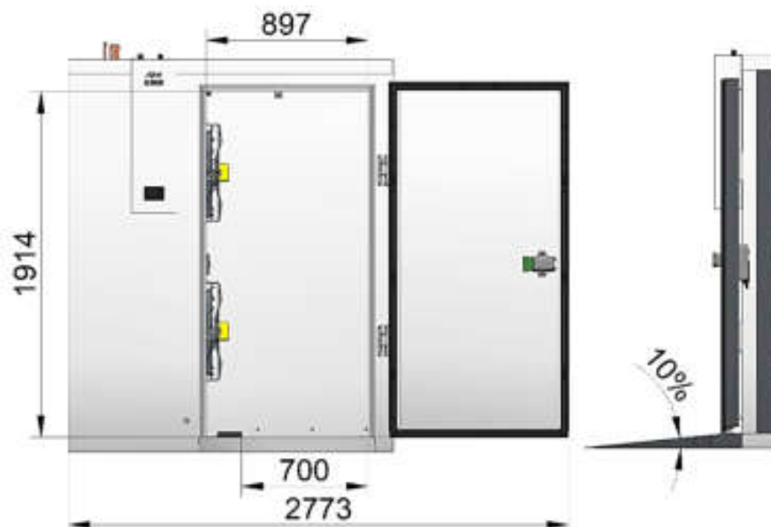
Рис. 7 Габариты входного проема камер
