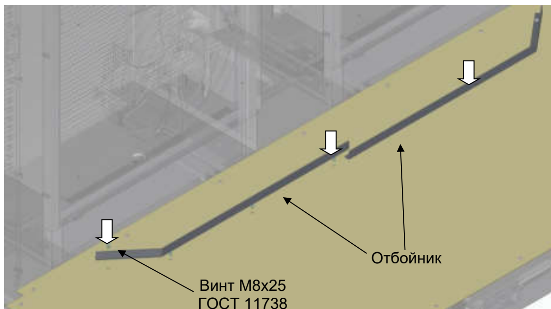
Рис. 26 Установка отбойника
