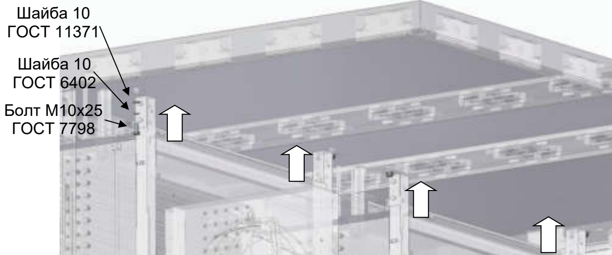
Рис. 20 Сборка крыши
