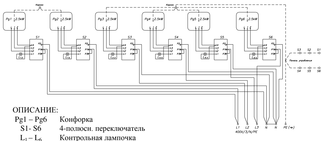
Рис. 2в: Схема электросоединений ES-T67/P и ES-T69/P
