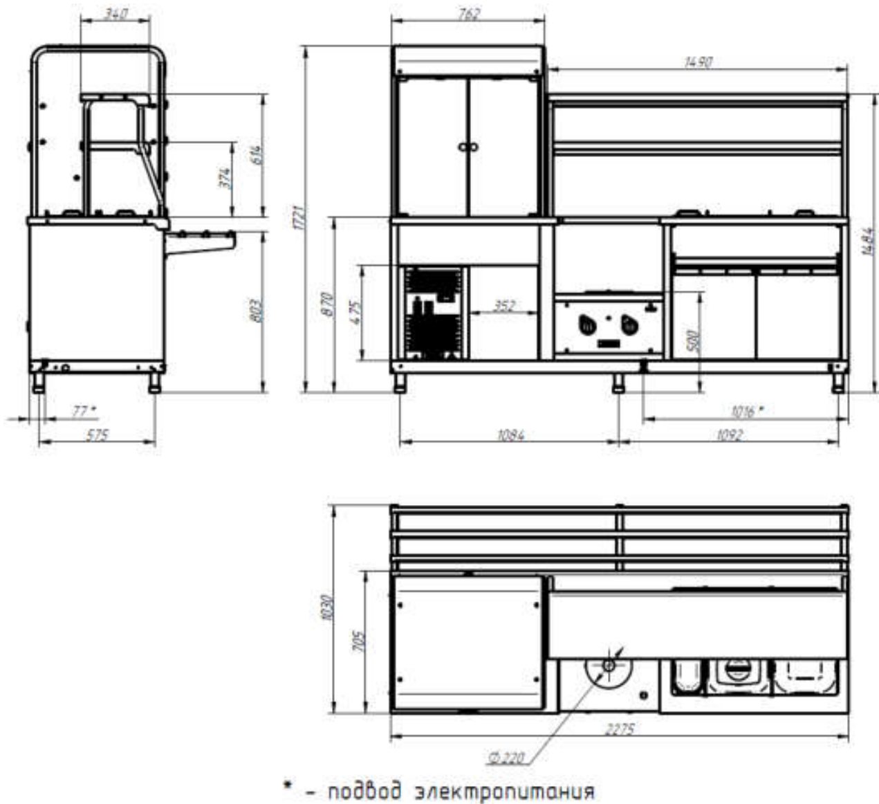
Рис. 1 Общий вид прилавка-витрины холодильной мармита PBXM-70KMU правый
