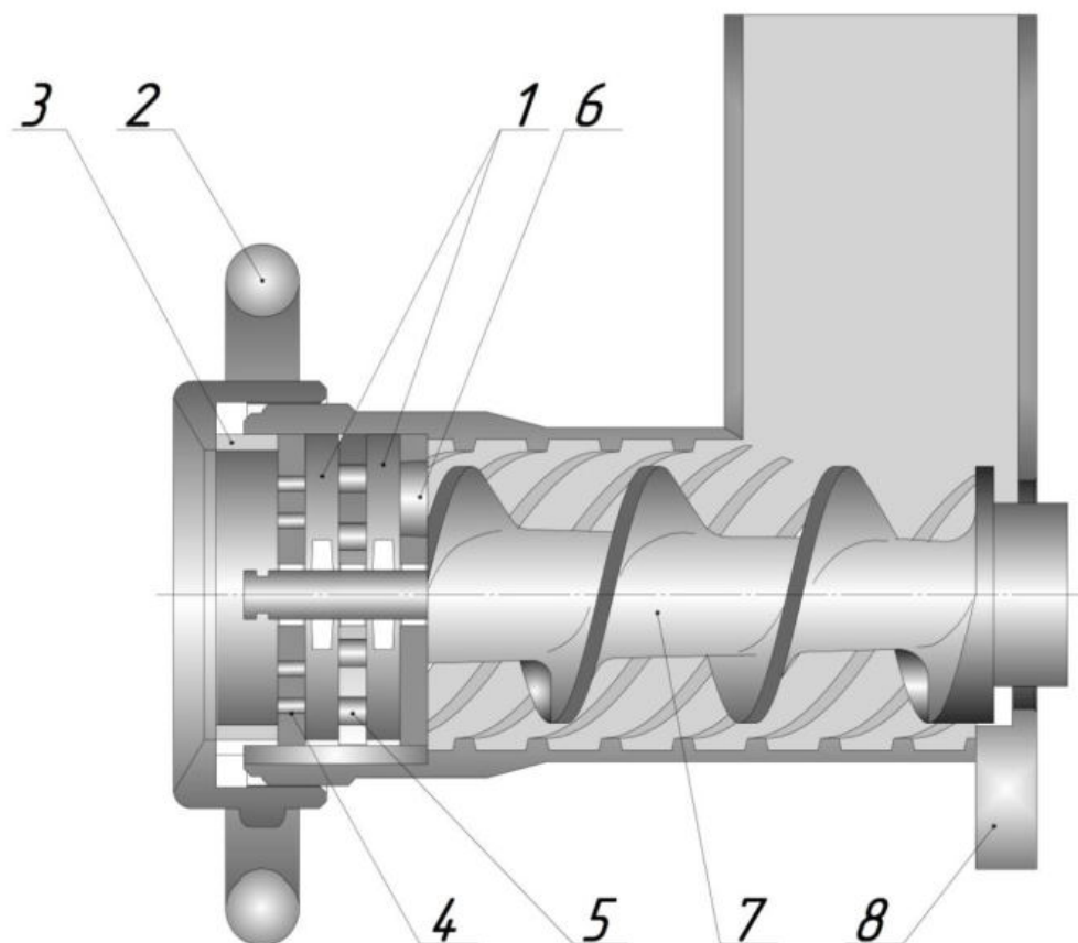
Рисунок 4 – Насадка - мясорубка
