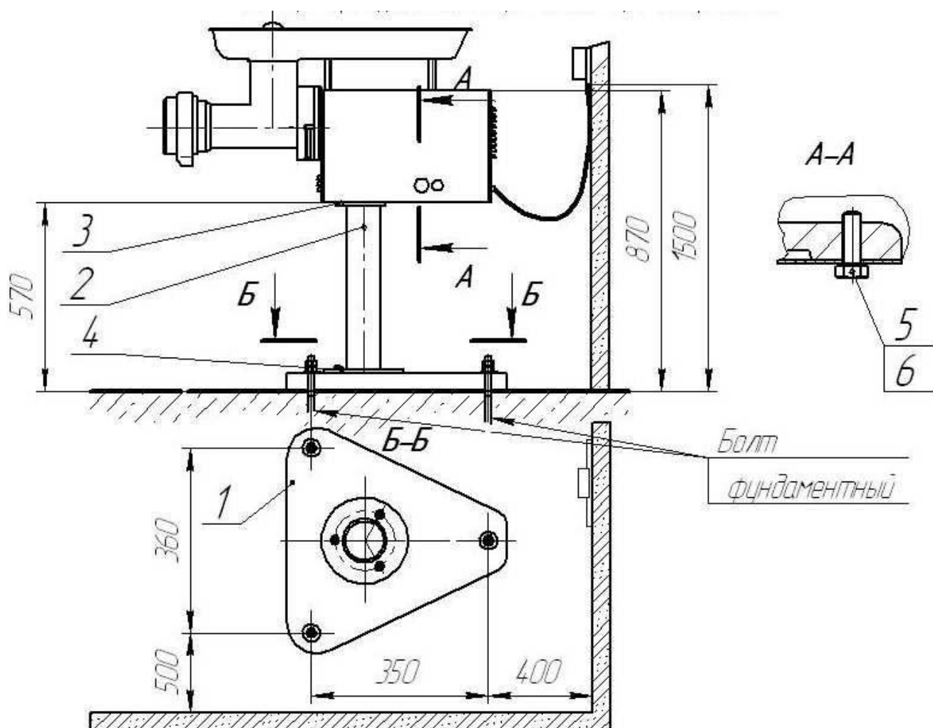
Рисунок 9 – Мясорубка М-600П
