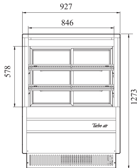
ВИД СПЕРЕДИ
