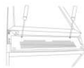
12. Namontujte spodní panel.
