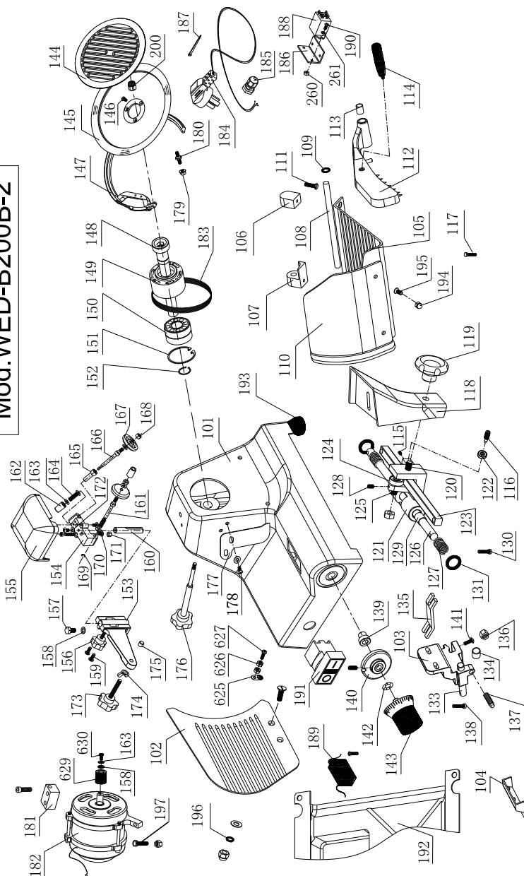
Рис.2 – Деталировка модели WED-B200B-2 (WED-B220B-2)
