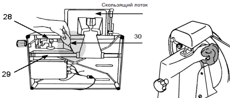
Рис. 7 – Очистка штока
