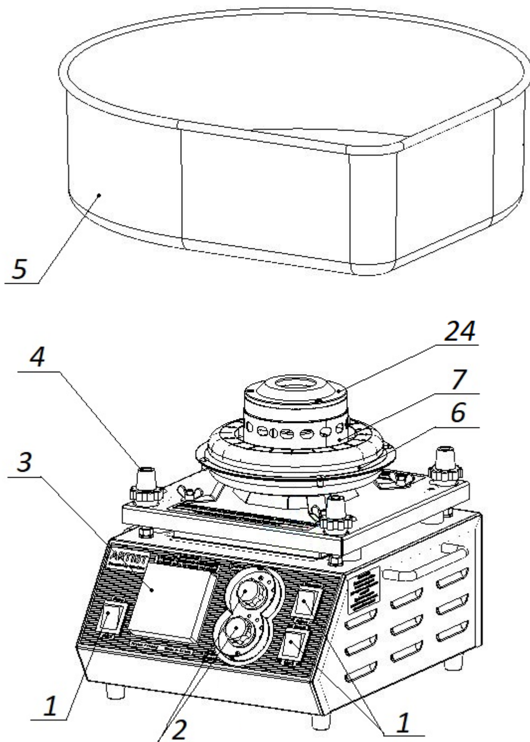
Рисунок 1 – Общий вид
