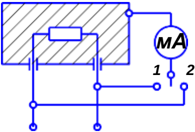
~220В Рисунок 2 — Схема измерения тока утечки
