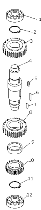
Рис. 3 – Детализовка. Приводной вал
