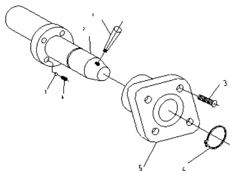
Рис. 5 – Переключатель скоростей
