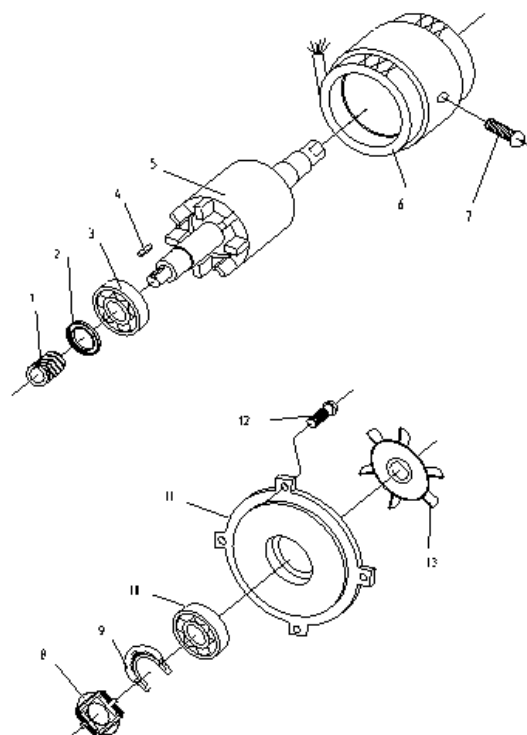
Рис. 4 – Деталировка. Электродвигатель
