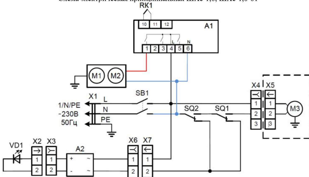
Перечень элементов ШХс-1,0, ШХс-1,0-01
