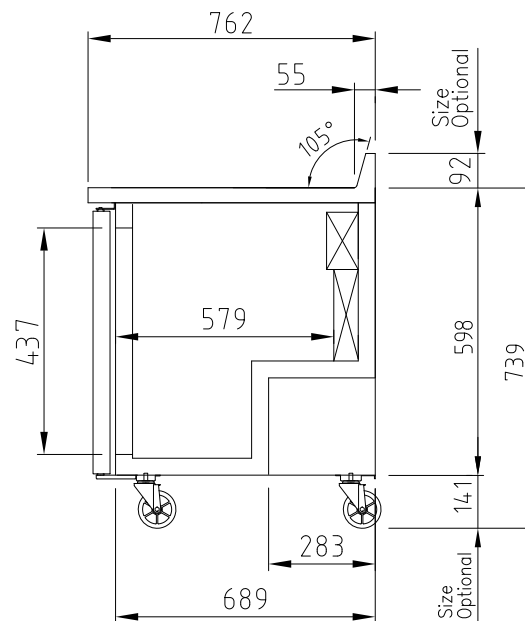
ВИД СБОКУ
