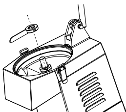
Рис. 9 – Очистка режущего лезвия (ножа)
