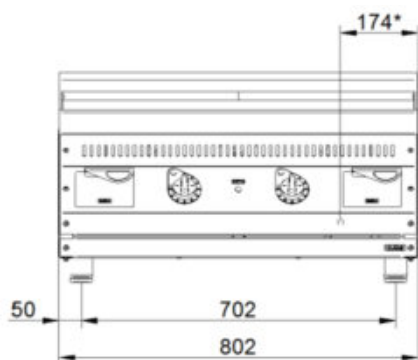
Рис. 3 - Общий вид ЭГЛ-80/2Н-00, где * - подвод электропитания
